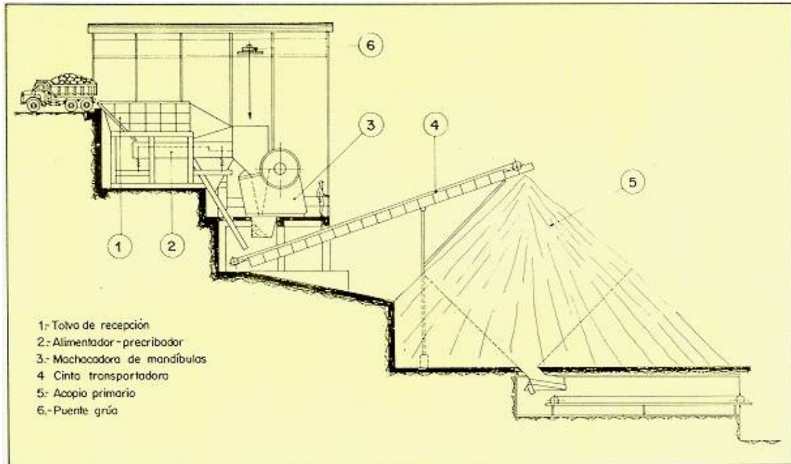
Fig. 2: Grupo primario de trituración
