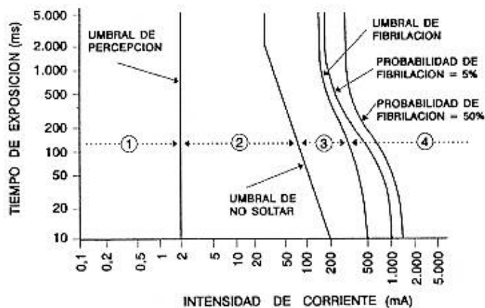
Fig. 11: Efectos de la corriente continua ascendente, en adultos, con trayectoria pies-mano izquierda
