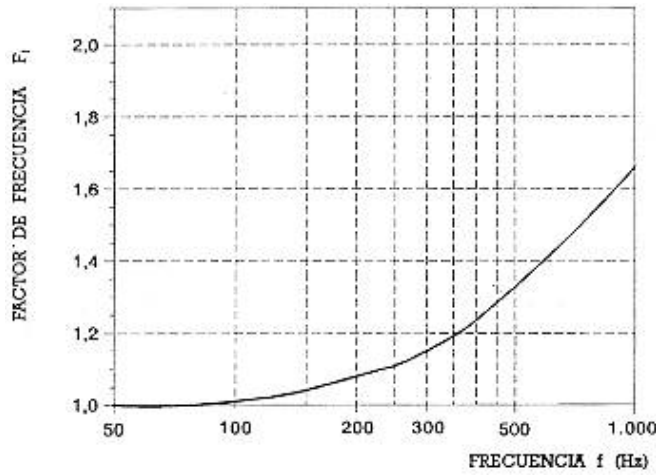
Fig. 4: Umbral de no soltar. F_f para frecuencias comprendidas entre 50 y 1.000 Hz
