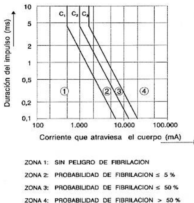
Zonas de peligro para la descarga de un condensador, para valores de 3T \leq 10 ms, para un trayecto mano izquierda-los dos pies
