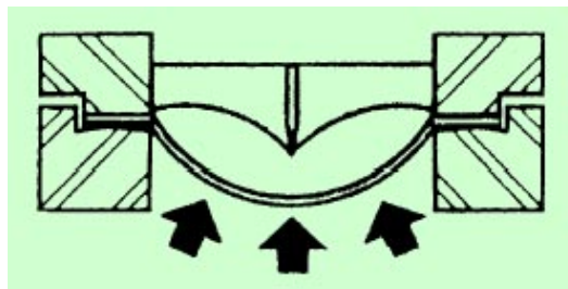
Fig. 3. Disco de ruptura abovedado invertido con hojas de cuchilla
